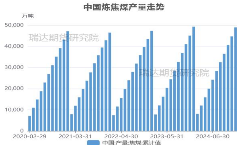
图18、炼焦煤产量
