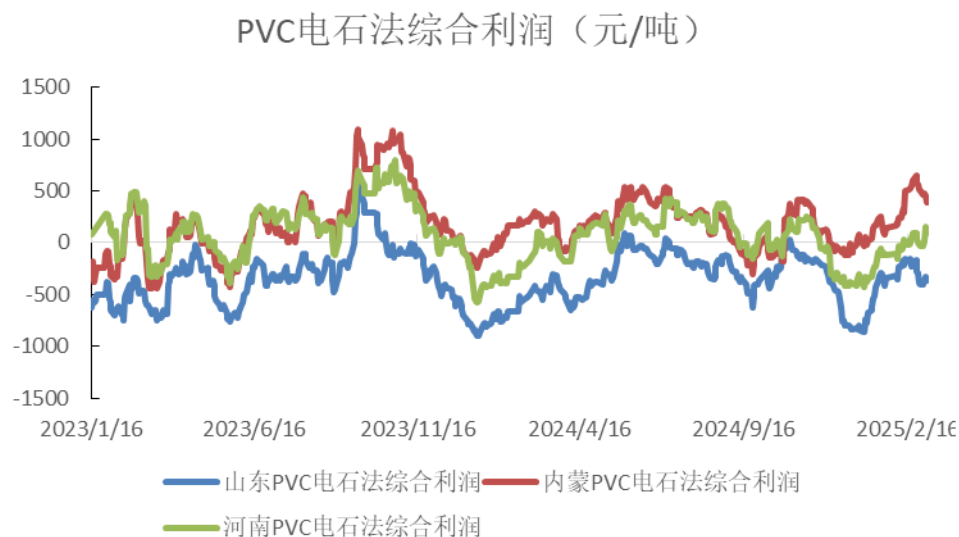
图33、聚氯乙烯 电石法利润
