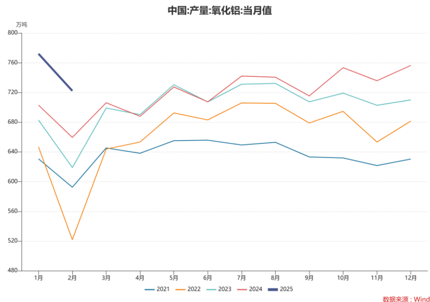
图18、氧化铝产量
