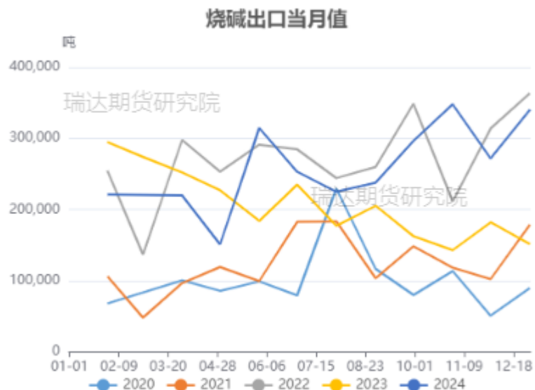
图26、烧碱出口量
