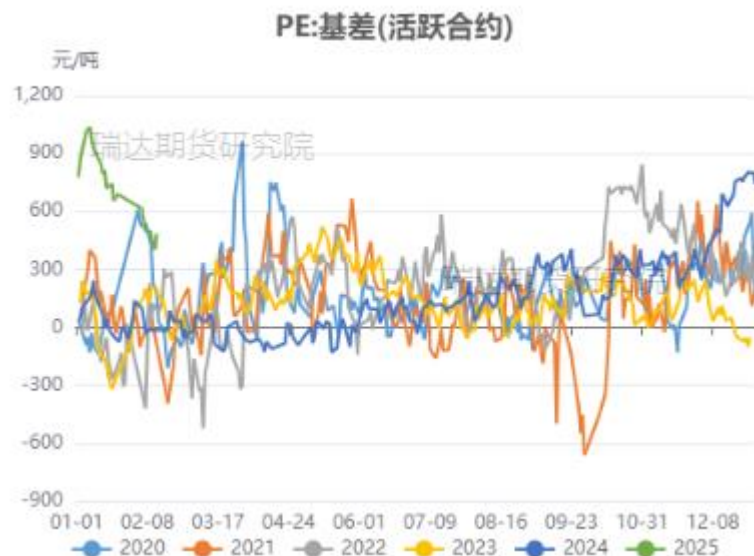
图11、聚乙烯基差
