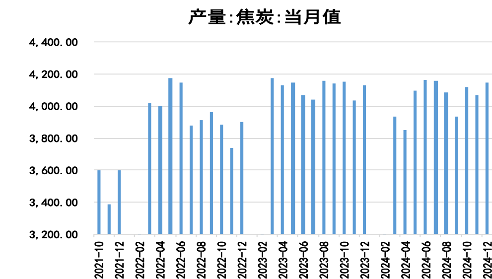
图10、焦炭产量
